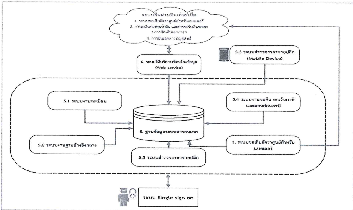
รูปแสดง แผนภาพรวมระบบที่จะพัฒนาและปรับปรุงในโครงการ
