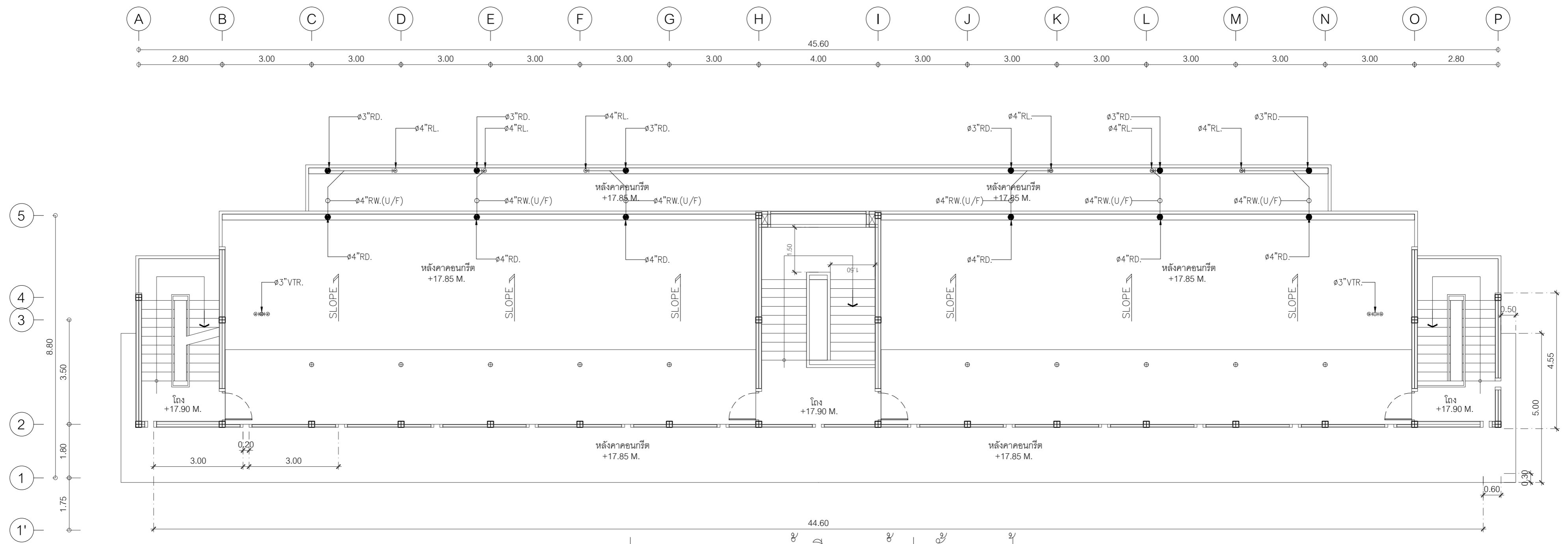
แปลนระบบระบายน้ำเสียและน้ำฝนชั้นดาดฟ้า มาตรฐาน 1:100
