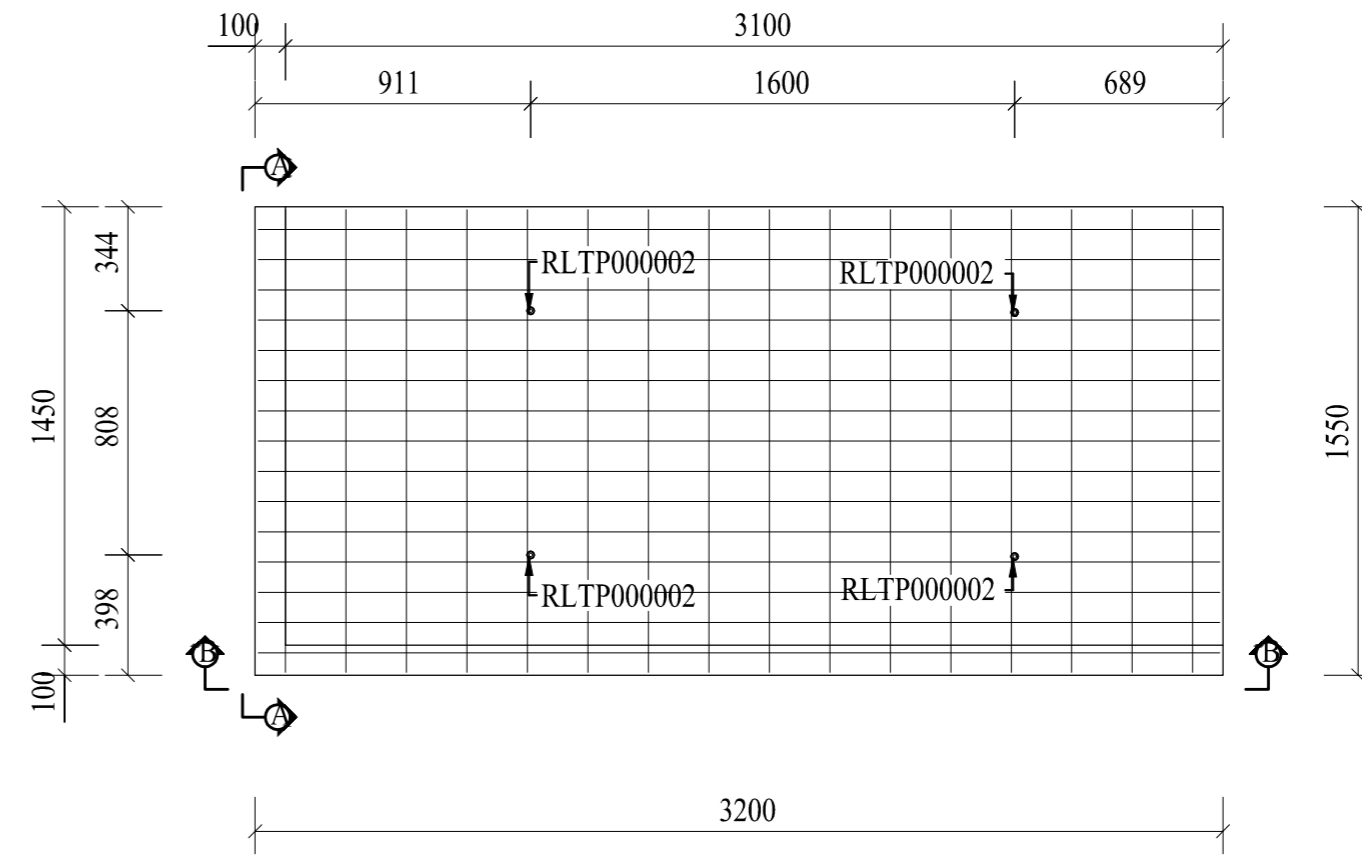
Plan (1:25)
