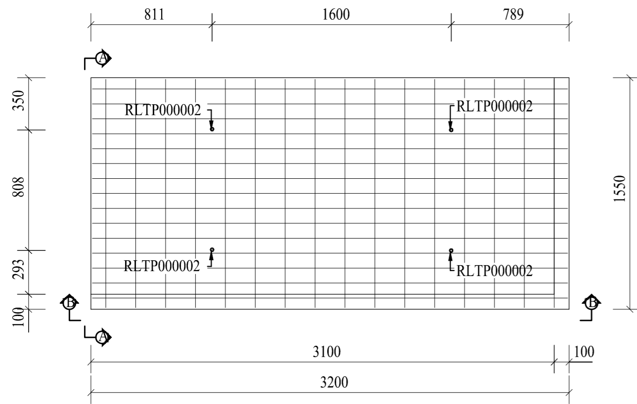
Plan (1:25)
