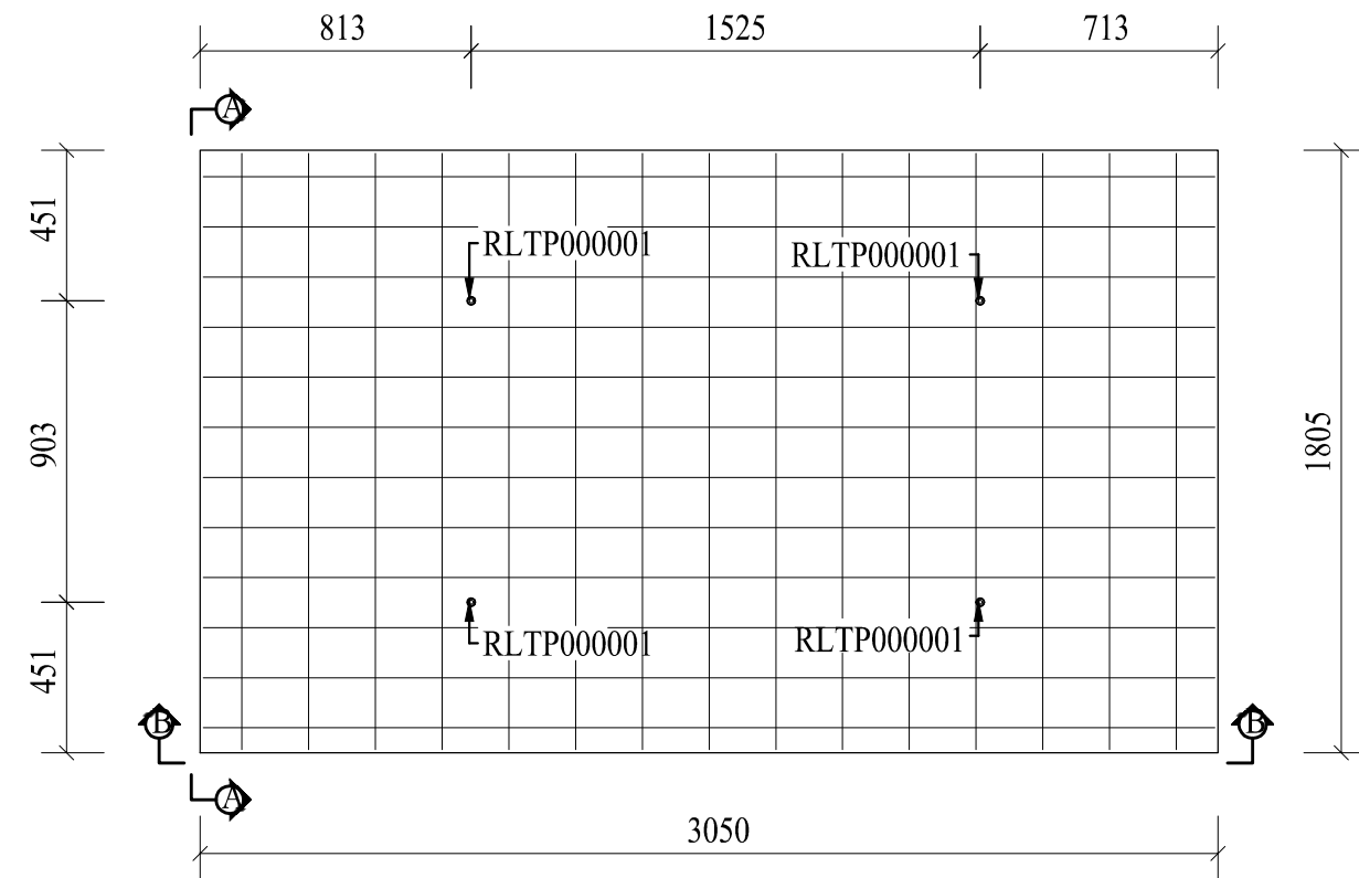
Plan (1:25)
