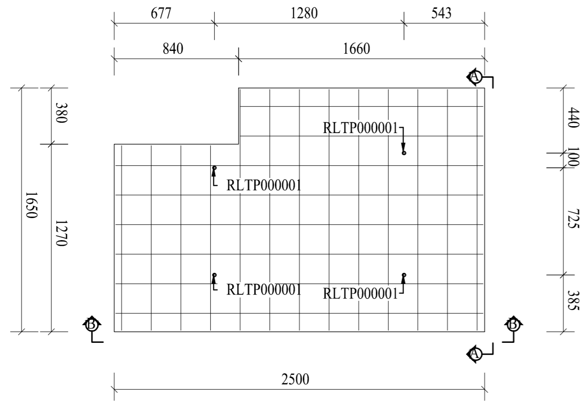
Plan (1:25)
