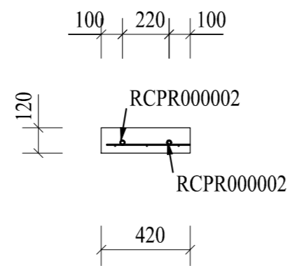
B - B (1:25)
