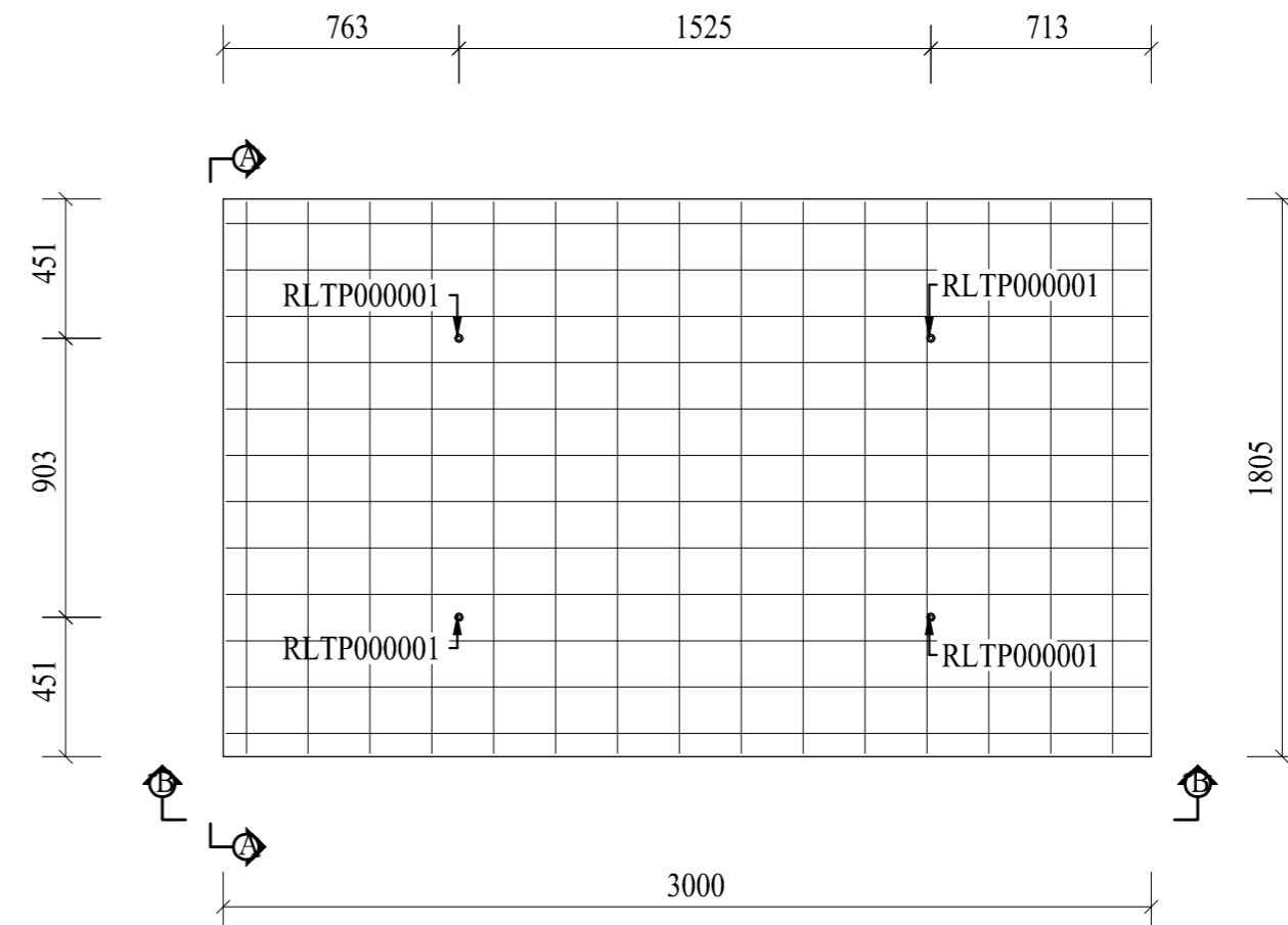
Plan (1:25)
