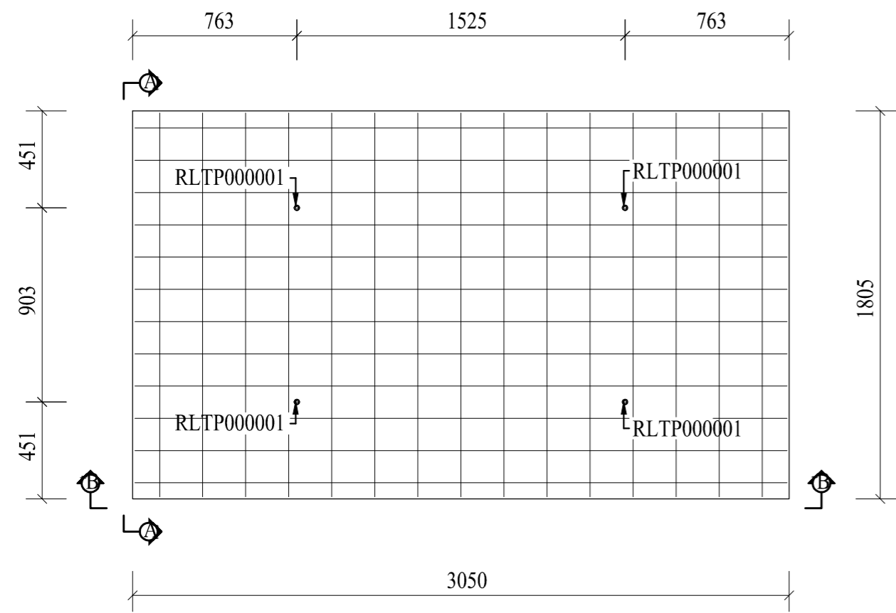
Plan (1:25)
