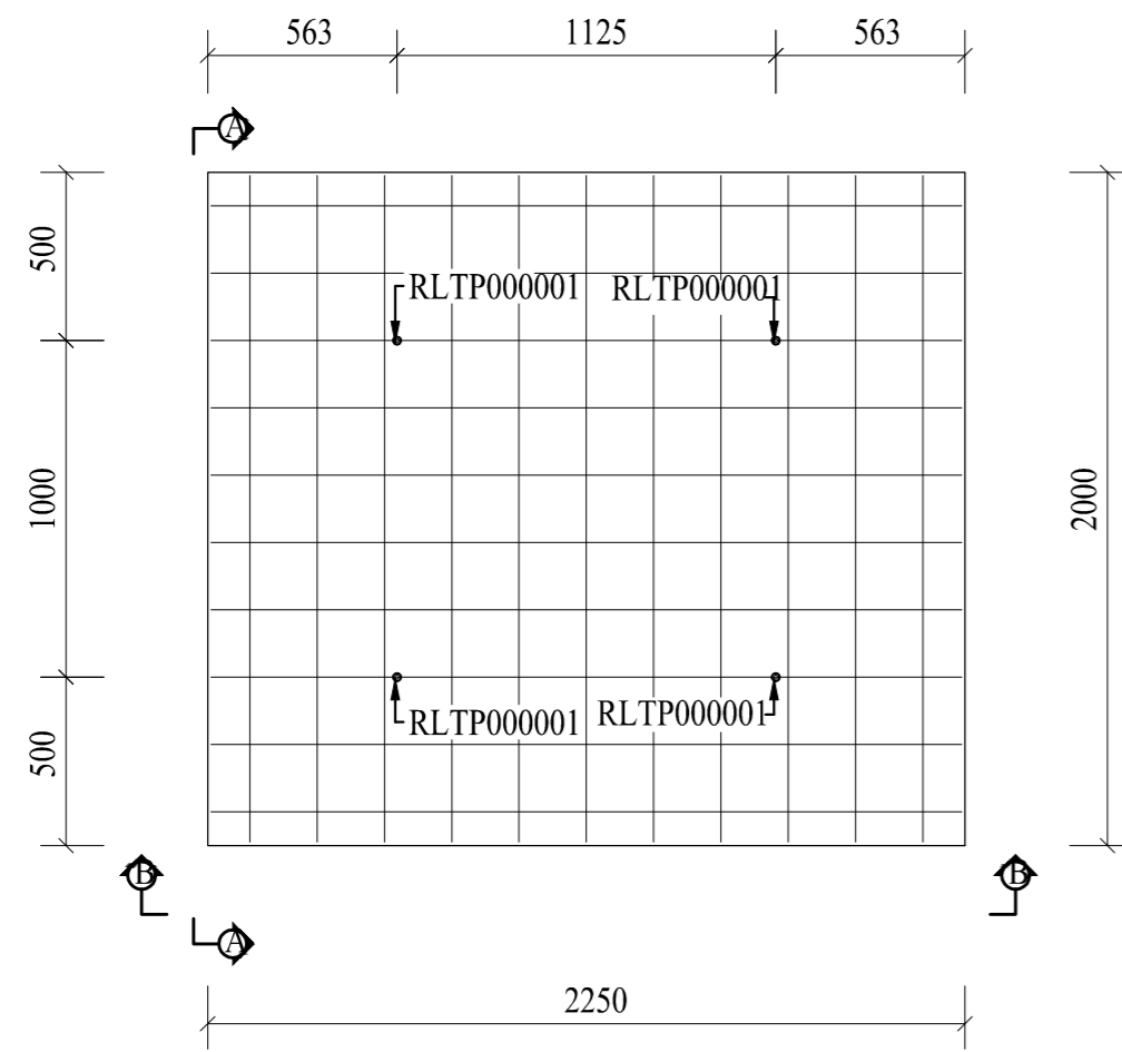
Plan (1:25)
