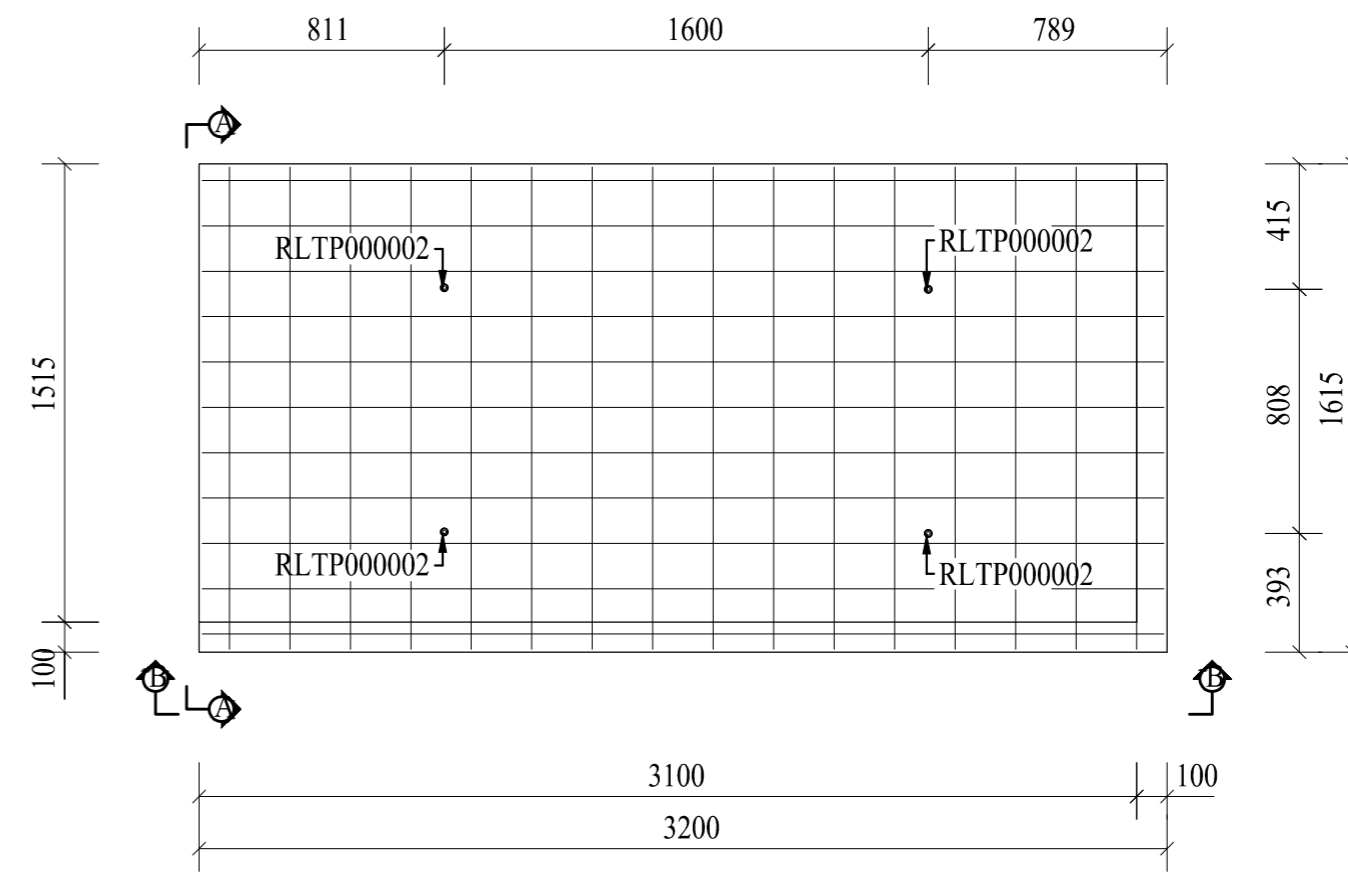
Plan (1:25)
