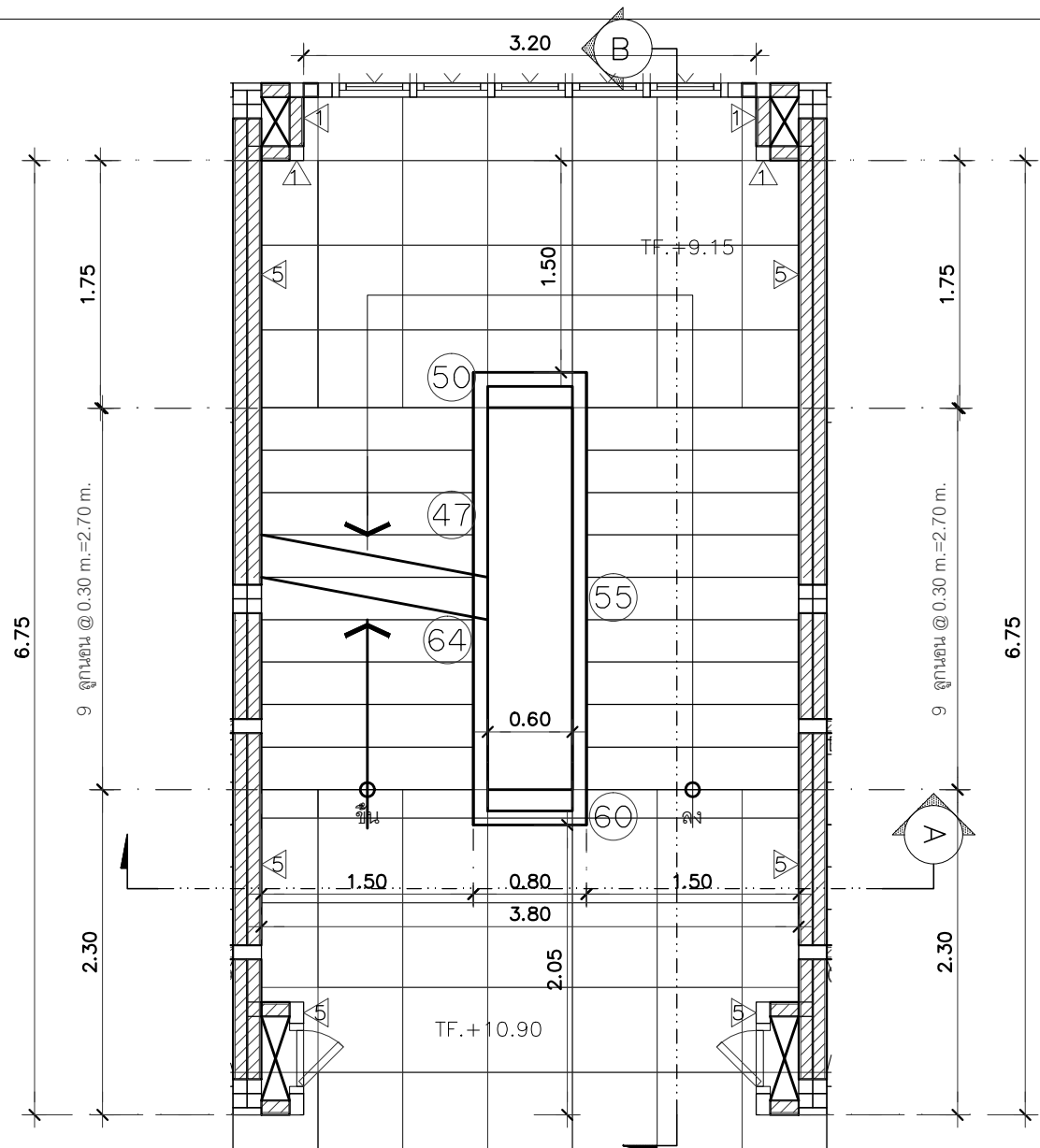
แปลนพื้นที่ 4th +10.95 SCALE 1:50
