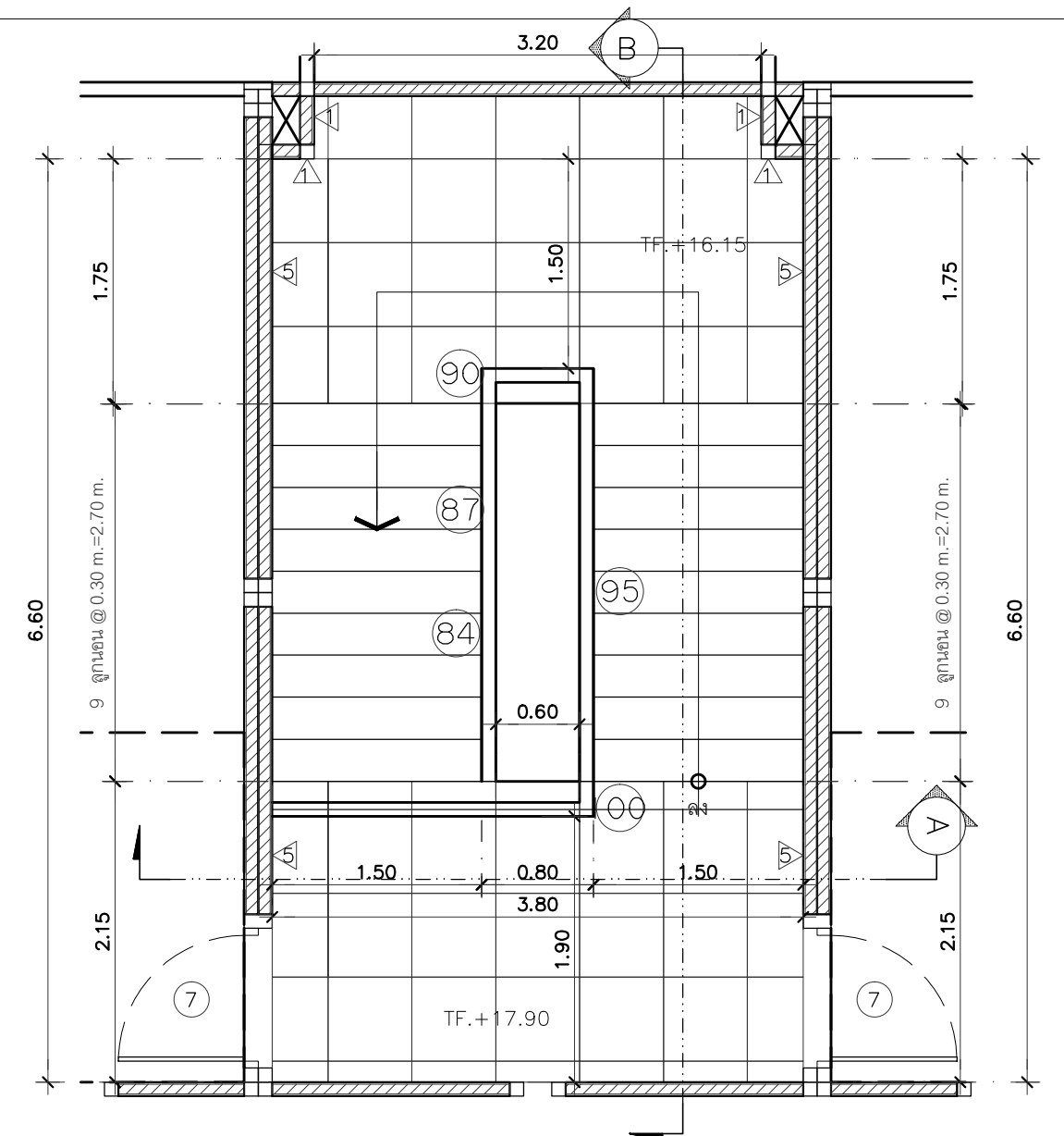
แปลนพื้นที่ 6th +17.90 SCALE 1:50
