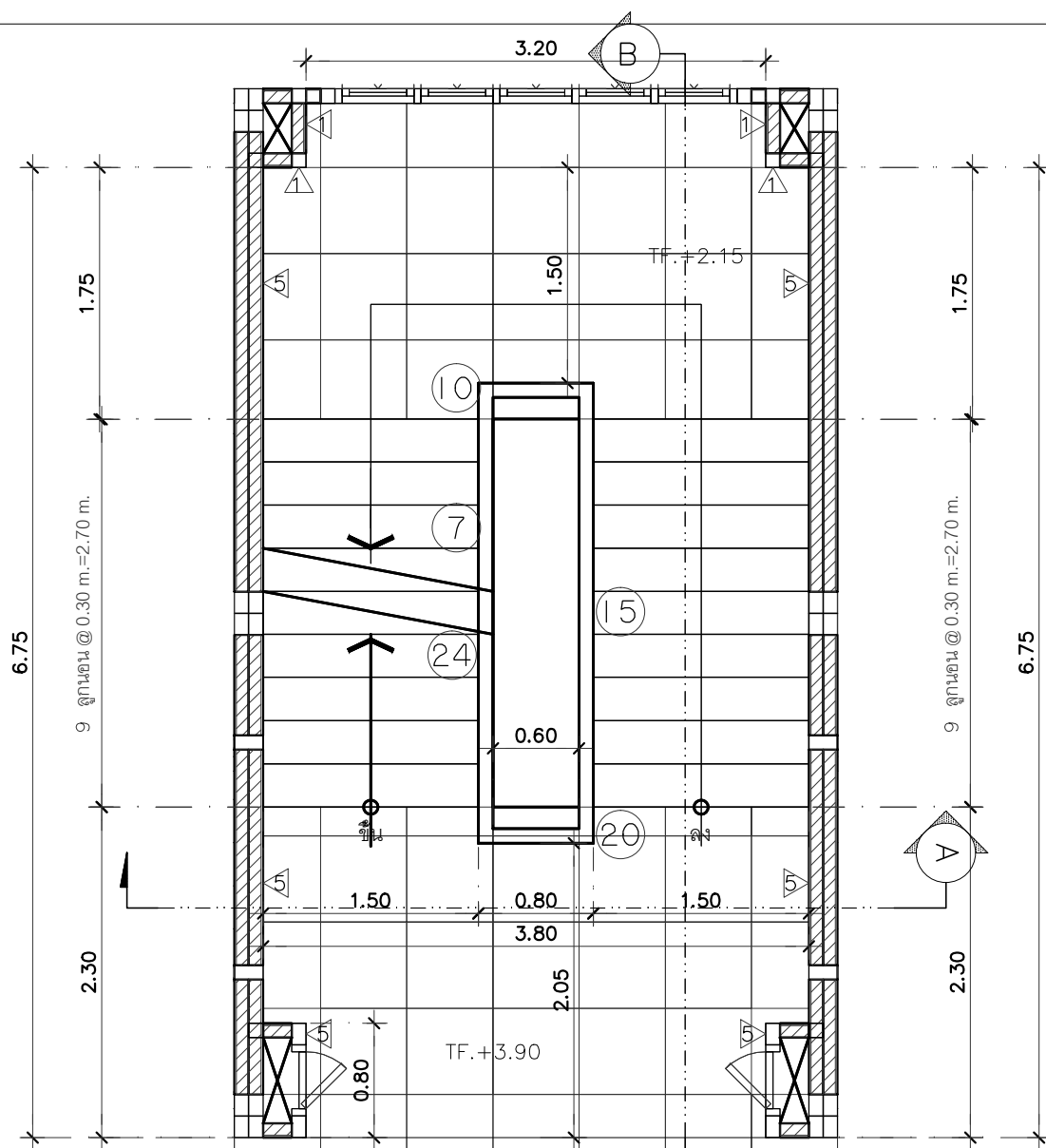
แปลนพื้นที่ 2nd +3.95 SCALE 1:50
