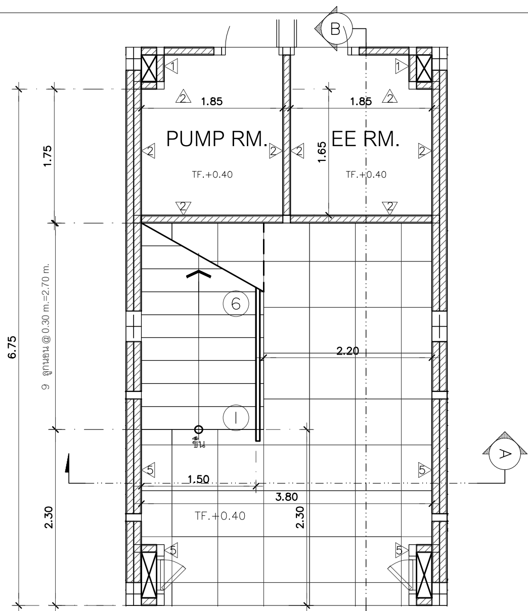
แปลนพื้นที่ 1st SCALE 1:50
