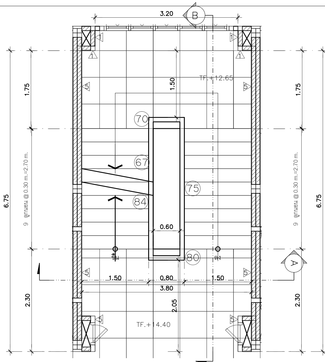
แปลนพื้นที่ 5th +14.45 SCALE 1:50
