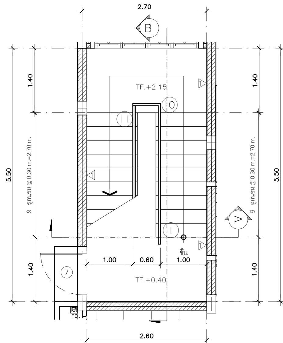
แปลนพื้นที่ 1st SCALE 1:50
