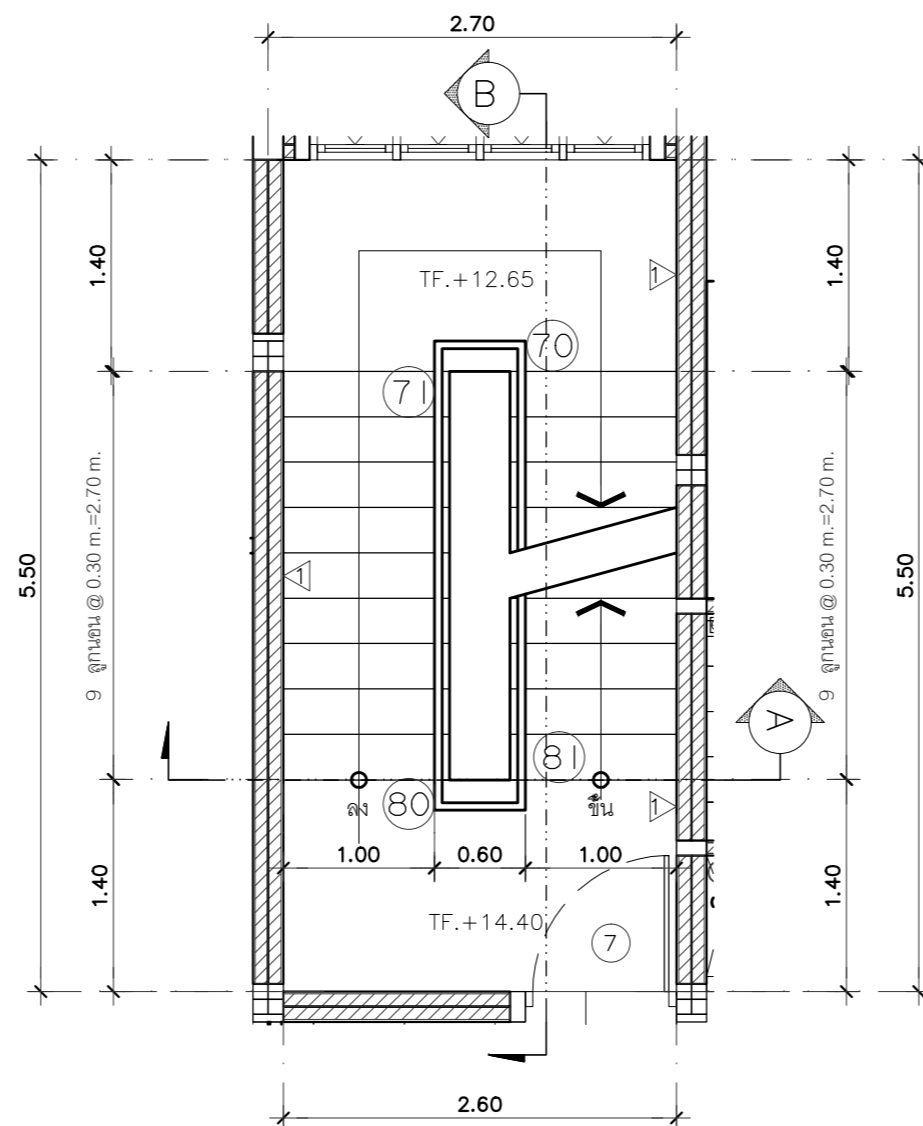
แปลนพื้นที่ 5th +14.45 SCALE 1:50
