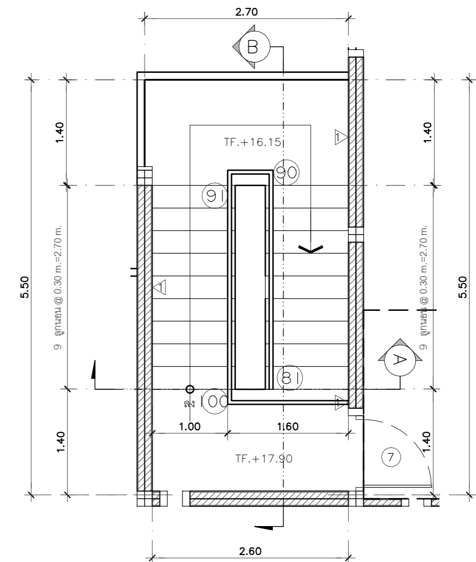
แปลนพื้นที่ 6th +17.90 SCALE 1:50
