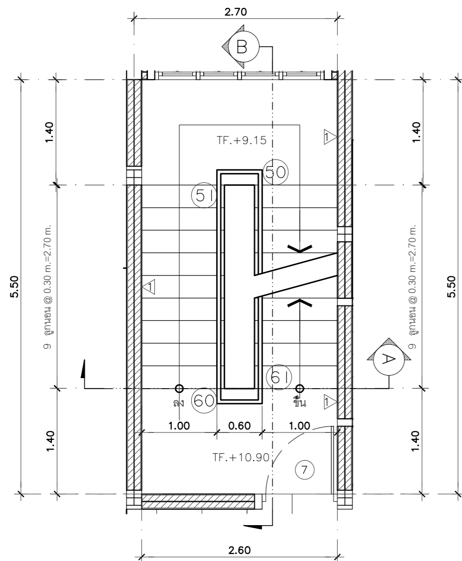
แปลนพื้นที่ 4th +10.95 SCALE 1:50
