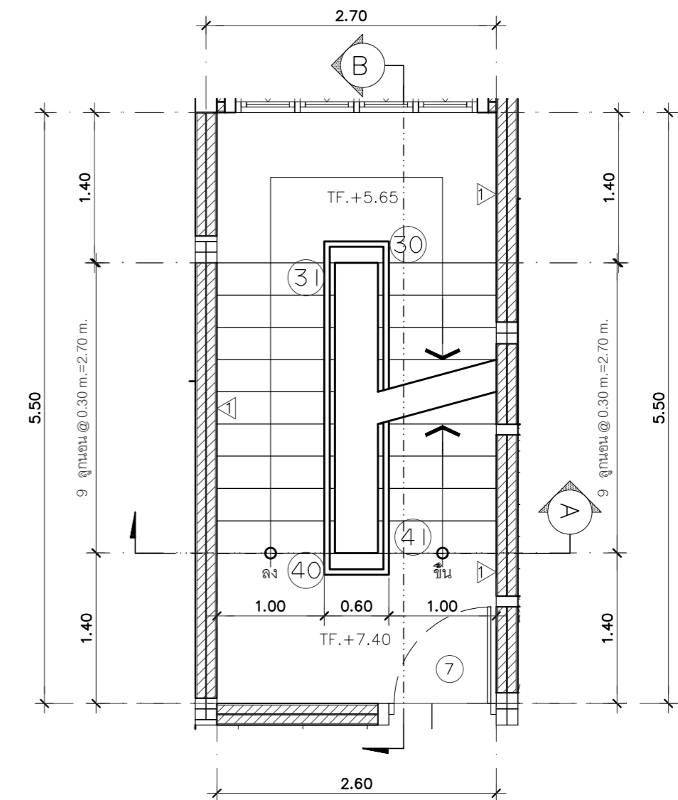
แปลนพื้นที่ 3rd +7.45 SCALE 1:50
