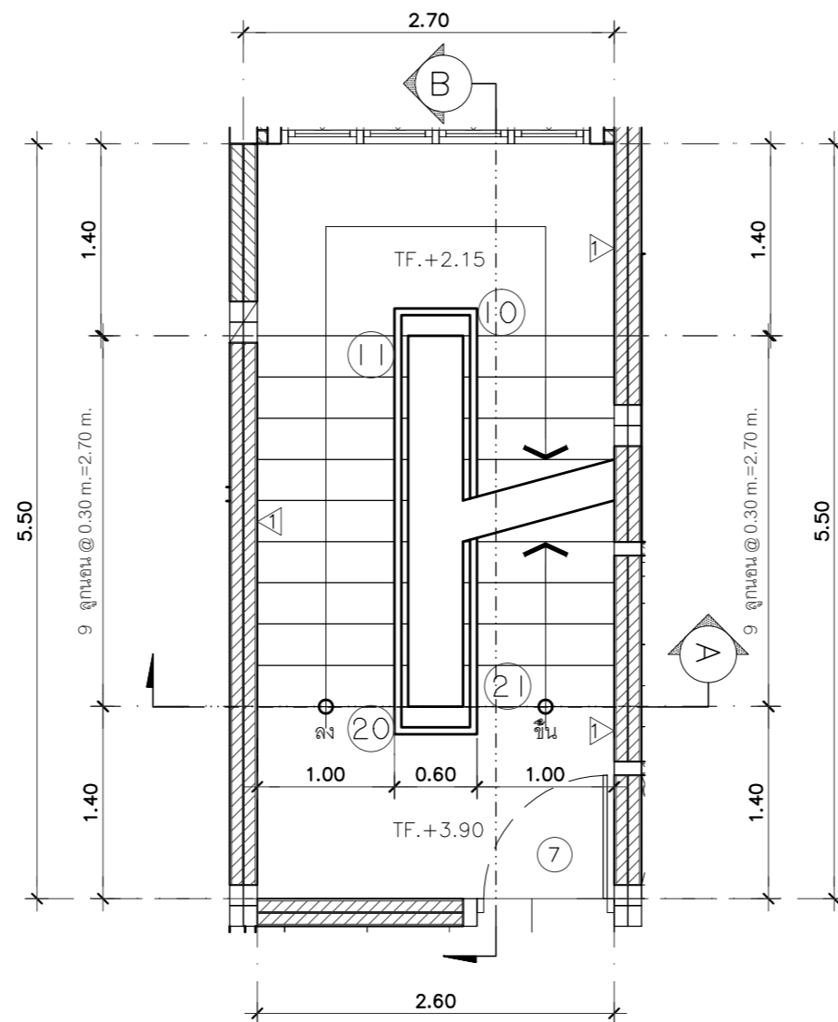
แปลนพื้นที่ 2nd +3.95 SCALE 1:50
